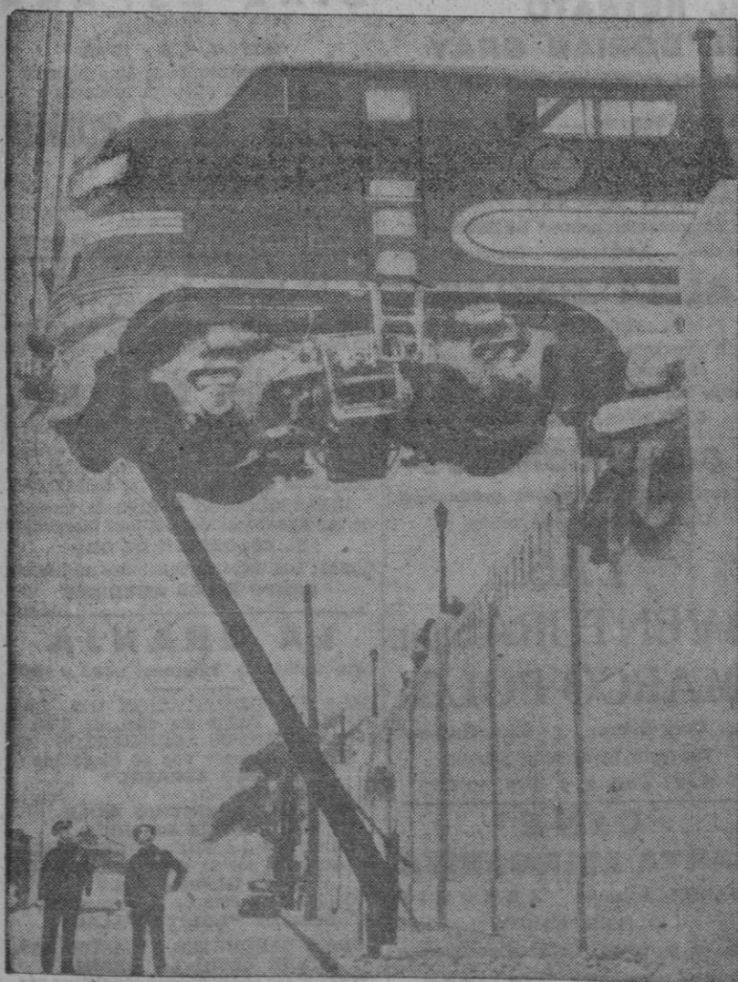
LOS ANGELES (CALIFORNIA).—Una locomotora, tipo Santa Fe, de un tren eléctrico, no pudo frenar a tiempo en la estación término, y quedó colgada en el espacio de esta forma espectacular que, gracias a un poste metálico y los cables de la electricidad, evitaron que el accidente revistiera caracteres graves.
