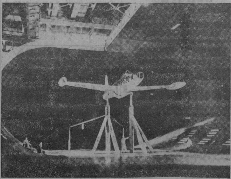
Prueba de las características de vuelo de un avión de reacción en el túnel aerodinámico supersónico en Moffett Field, en el Estado de California
