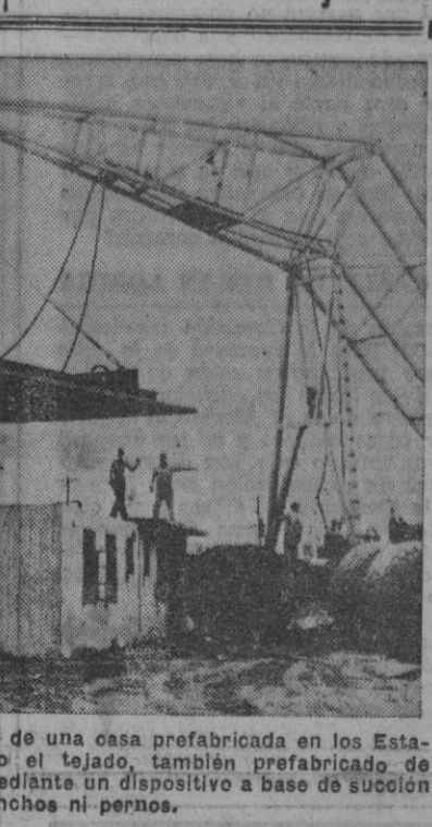
Durante las obras de construcción de una casa prefabricada en los Estados Unidos, una grúa coloca en su sitio el tejado, también prefabricado de hormigón, de 17 toneladas de peso, mediante un dispositivo a base de succión de aire, que no precisa el empleo de ganchos ni pernos.
