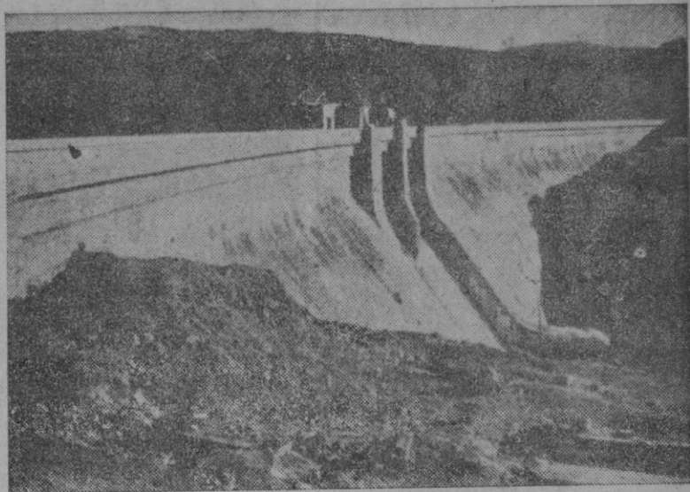
LA PRESA DE LAS CONCHAS, VISTA DESDE AGUAS ABAJO
