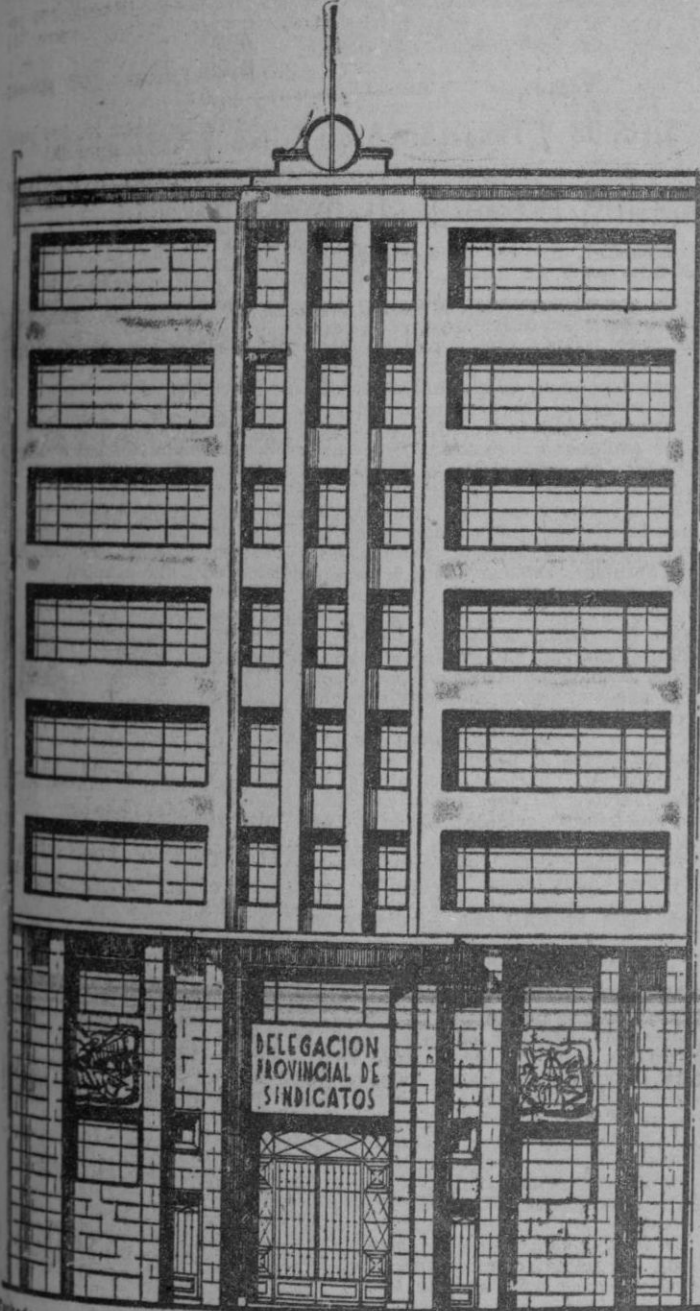
Edificio principal, a la calle de Pardo Bazán, del proyectado edificio de la Casa Sindical de La Coruña
