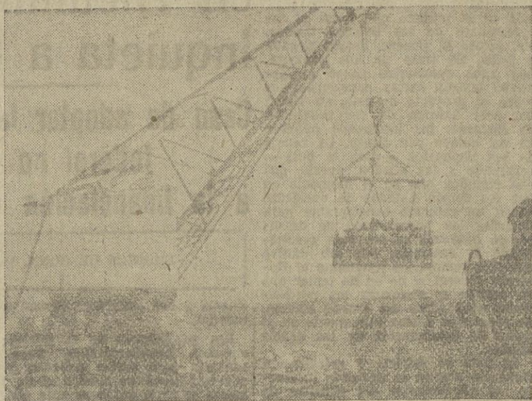
La grúa mantiene suspendida de su pluma un cargamento de ocho toneladas de piedra que luego depositará en el lugar preciso. Es la misma vagoneta, cuya parte superior se separa del carro y sobre el que luego vuelve a colocarse.
