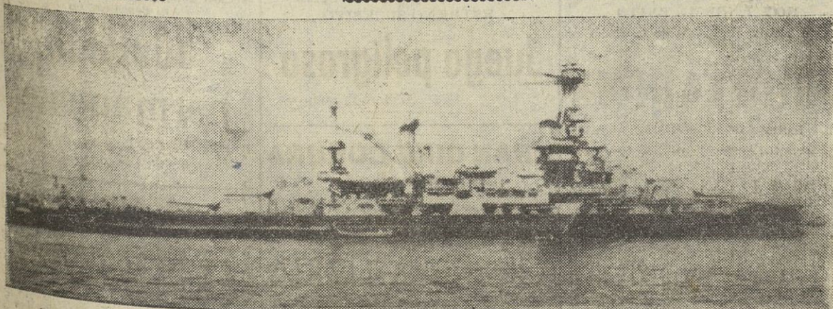
El acorazado "Lorraine" de 166 metros de eslora, 27 metros de manga y 8,50 de puntal con 20.900 toneladas de desplazamiento, que ha sido puesto en venta en Tolón, pero que no ha sido vendido porque ninguna oferta ha alcanzado el precio mínimo fijado por la Administración. Parece ser que este mínimo sería de 200 millones de francos y que será aplazada su venta tres meses
