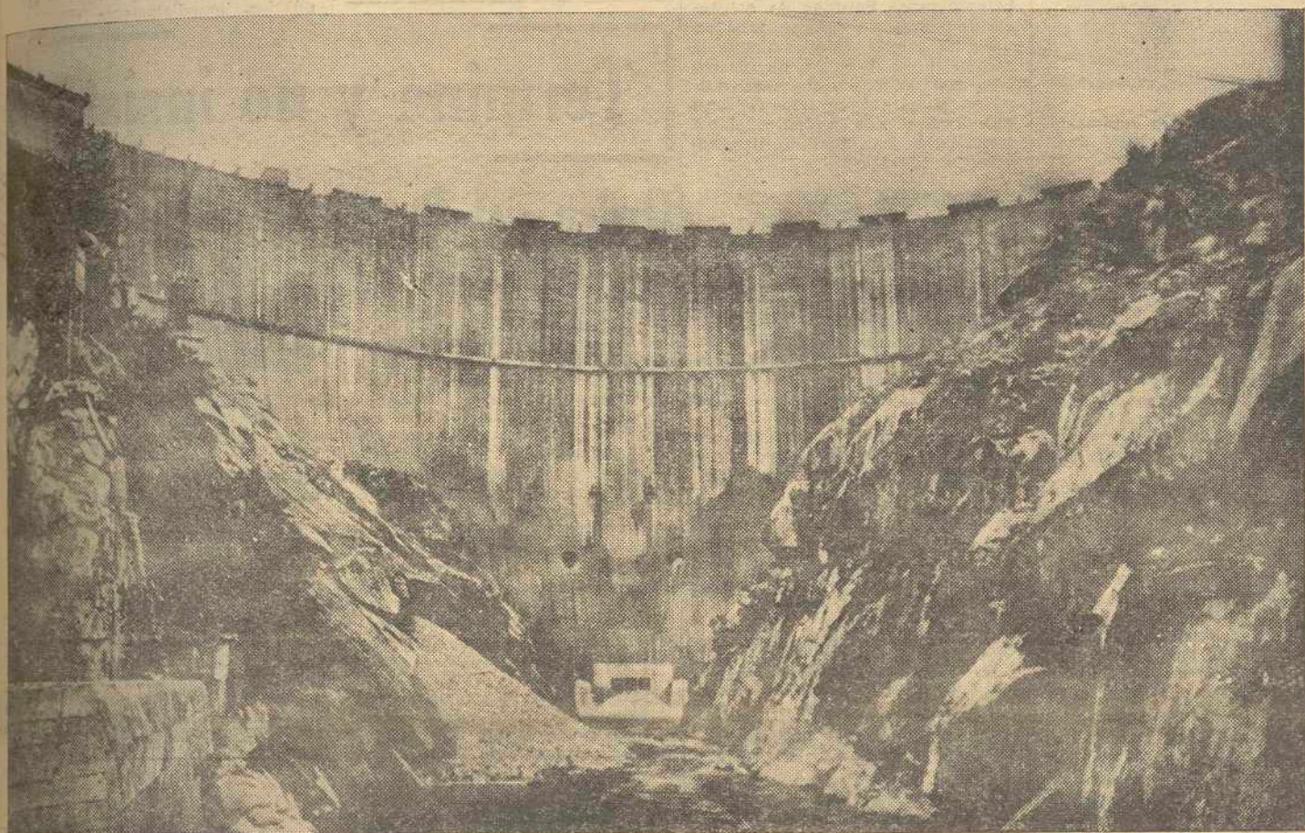
VISTA DE LA PRESA DESDE AGUAS ABAJO
