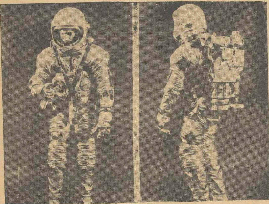
HOUSTON (Texas). — He aquí los prototipos de trajes espaciales para el proyecto "Apollo" a la Luna, los cuales han sido revelados por el centro espacial de Houston, Texas. La goma de los brazos, piernas y torso facilitan una gran movilidad. El traje permite comer y beber en pleno espacio o en la Luna. El aparato de la espalda provee al astronauta de oxígeno, ventilación control de temperatura y humedad y renueva la atmósfera del interior del traje. — (Foto EUROPA PRESS)
