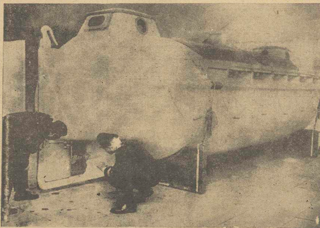
FRANKFURT. — Se han efectuado con éxito las primeras pruebas del submarino «Tiger-shark», para dos personas. El prototipo ha tenido un costo de 25.000 marcos. Tiene una velocidad de crucero en superficie de 10 kilómetros horas y siete de inmersión. Lo mueve un motor eléctrico de 2 HP. La producción en serie de este pequeño submarino deportivo comenzará en junio de este año con el lanzamiento de docenas unidades. — (Foto EUROPA PRESS)
