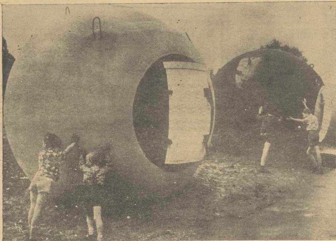
HAMBURGO. — Estos refugios esféricos, transportables, de hormigón armado contra bombas atómicas, pesan 5.5 toneladas cada uno. Su precio es de 6.900 marcos (1.720 dólares). Para su instalación interior se tendrán que gastar otros 3.000 marcos (750 dólares). Se puede colocar la bola en cualquier sitio al aire libre, donde hay que amarrarla. También es posible enterrarla hasta la parte inferior de la puerta, incluso junto al sótano de la casa, de donde, por medio de una abertura en la pared, se podrá entrar directamente en la "bola antiatómica".
