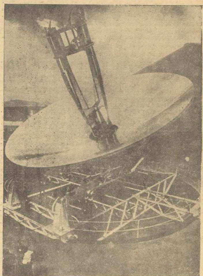
Un espejo plateado de 45 pies de diámetro ha sido instalado en Denver, Colorado, para convertir en energía eléctrica los rayos solares. Su foco puede producir temperaturas superiores a los 2.000 grados. — (Foto AP-LOGOS)
