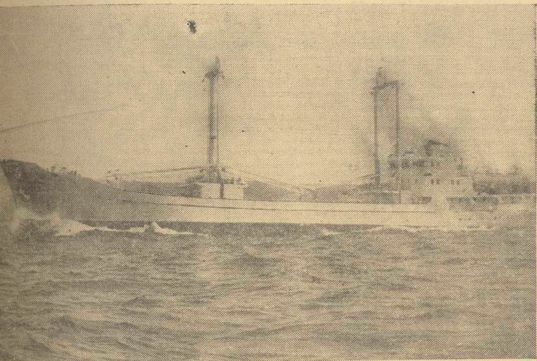
Recientemente fué botado en Perillo el «Glaciar Azul», que aparece en nuestro grabado realizando las pruebas de mar en aguas de la mundialmente famosa ría ferrolana. Este buque, que forma parte de una serie que construye ASTANO, será dedicado al transporte de fruta. Desplaza tres mil toneladas. — Foto BERNARDINO
