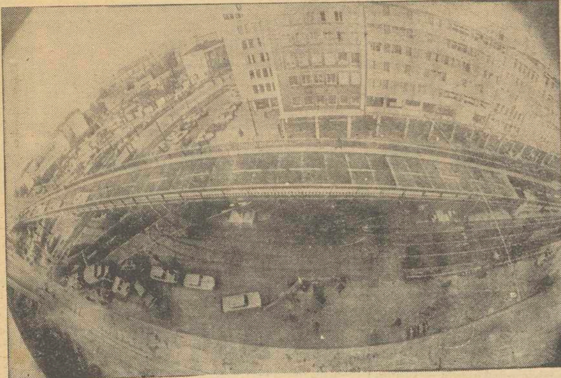
El nuevo viaducto levantado sobre la Plaza de la República en Frankfurt del Meno (Alemania), presenta una forma elipsoidal visto a través del objetivo de una "cámara de ojo de pez" que permite un ángulo visual de 180 grados. Con ello la foto da una idea completa del viaducto más moderno de Alemania.— (Foto-Fiel).
