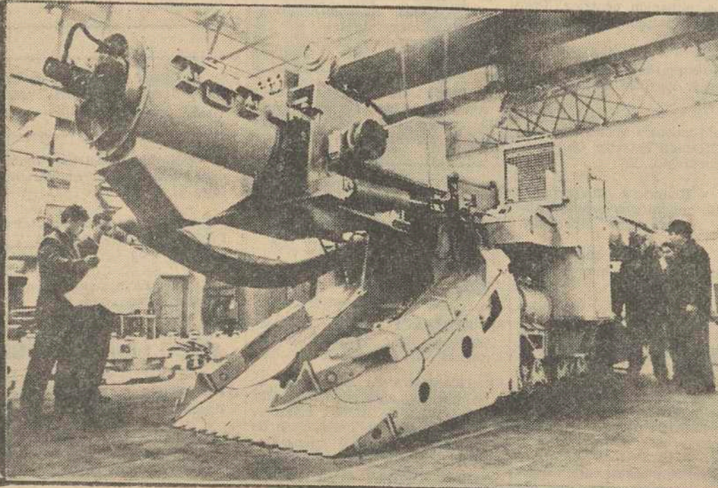
Científicos ucranianos acaban de construir un modelo experimental de un aparato que se piensa utilizar para destruir rocas y que podría llamarse... por ejemplo, "lanza-agua". Bien, pues el nuevo artificio dispara cada tres o cuatro segundos una descarga de 1,2 litros de agua contra la roca. La fuerza del choque es tan grande, que ésta, por muy dura que sea, queda destruida. Al parecer, el "lanza-agua" tendrá aplicación no sólo en minería, sino también en todo tipo de demoliciones. (FOTOFIEL)
