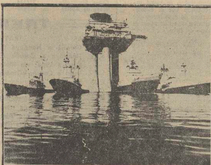
Esta es la nueva plataforma "Beryl A" que la Compañía Mobil Oil acaba de construir en Stavanger (Noruega). Es la primera de una nueva generación de estructuras de hormigón de 350 toneladas, y sostenida por tres columnas. Será utilizada para la extracción de petróleo destinado a Gran Bretaña. — (FOTOFIEL)
