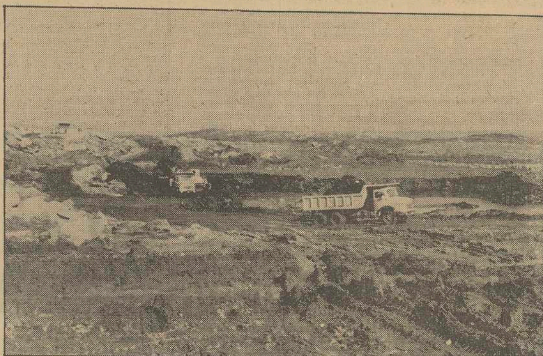
La fotografía recoge un aspecto de la zona de explanación de terrenos para la ubicación de la factoría de Alúmina, entre Llieiro y Bideiros, así como —a la izquierda— los trabajos intensos de las modernas máquinas perforadoras que intervienen en la metódica labor previa a las voladuras que siguen realizándose en el monte Saíñas. — (Foto SISO)
