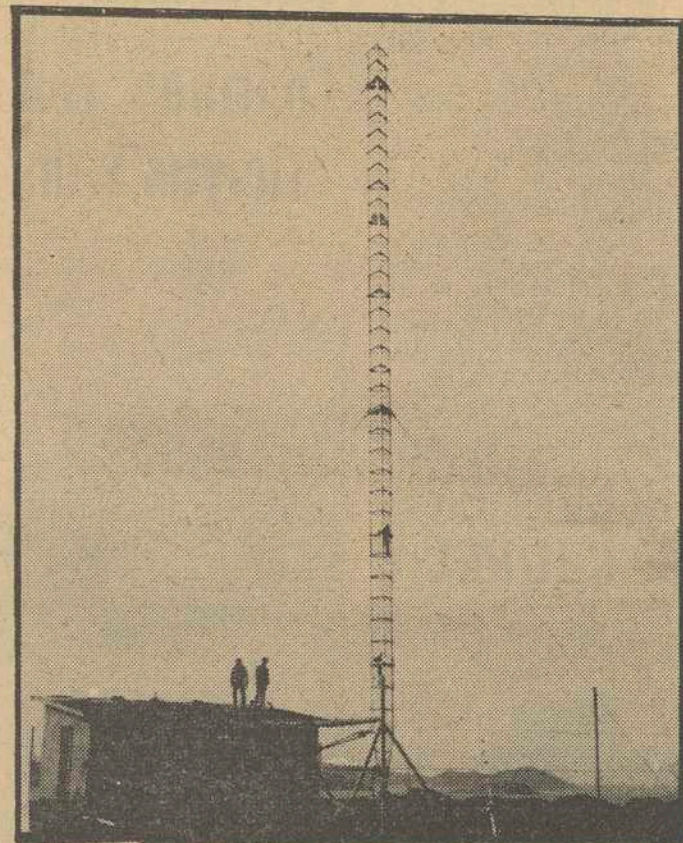
Un aspecto de la torre meteorológica que la Unión Central de Regadela está construyendo en el monte de la Cantera en la parroquia de Villachá. Lleva 42 metros de altura e irá equipada con diferentes aparatos de medida para la zona
