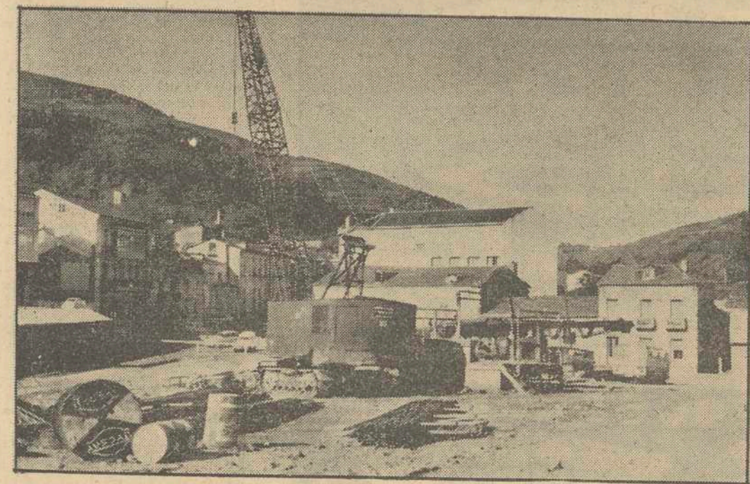
La fotografía muestra dos de las grandes máquinas que intervenían en los trabajos de la variante de Becerreá y que han sido desmontadas para su traslado a otra provincia. La del fondo es una singular máquina de pilotaje sin cuya intervención no sería posible la terminación de la obra en el corto plazo que tenían previsto. — (Foto SISO)
