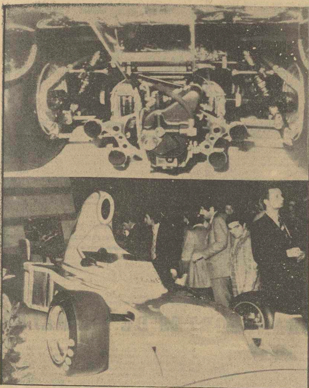
El "Ligier" nuevo bolido para el año próximo. En la foto de la parte superior podemos ver un detalle de su motor matra de 12 cilindros en V. Las pruebas de laboratorio que se han realizado con el mismo son óptimas, ahora falta enfrentarse con la realidad de la pista, que es lo principal. (Foto EFE-FIEL)
