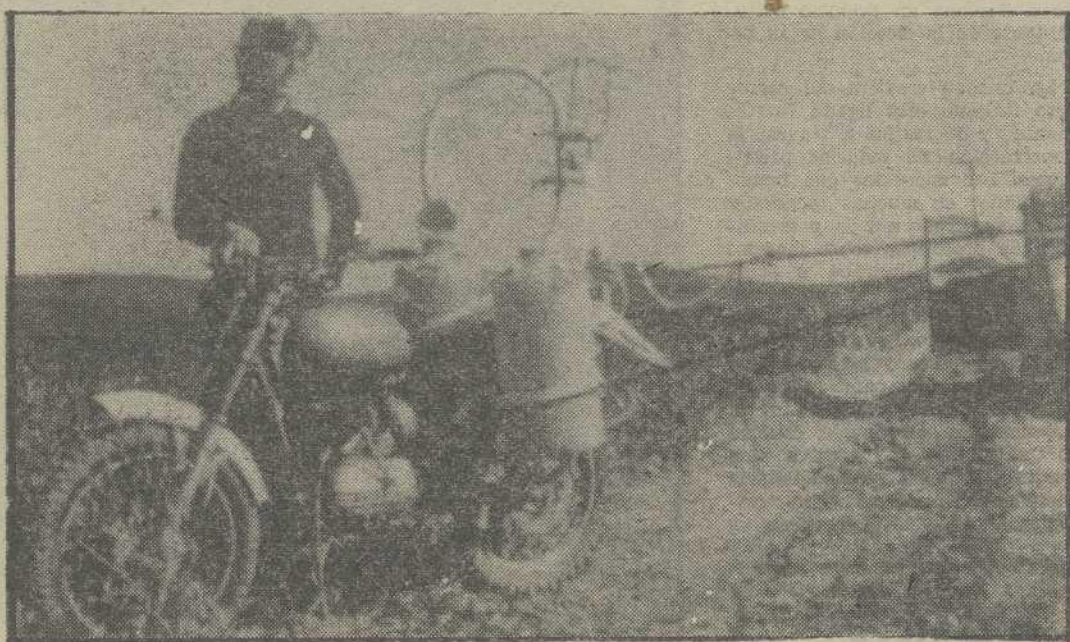
Tres hermanos de Marchena, Sevilla, han ideado un sistema que sustituye ventajosamente al tractor en los trabajos de reparto de herbicidas e insecticidas. Se trata de un bastidor acoplable a una motocicleta. Mientras las ruedas del tractor aplastan y destruyen muchas plantas sembradas, la moto puede circular con mayor facilidad por la parte baja de los surcos. — (Foto EFE-FIEL)
