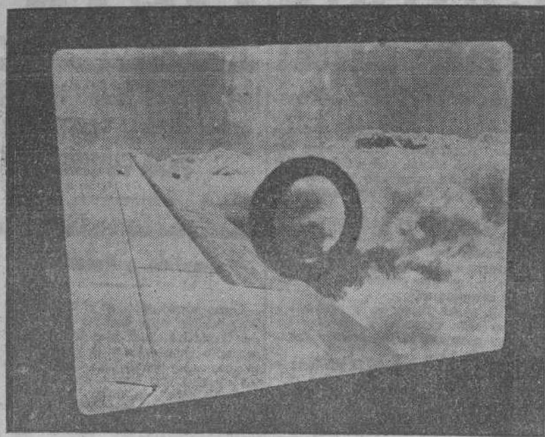
Este agujero en la ventanilla de un avión transporte americano, que lleva provisiones a través de las montañas del Himalaya, desde la India a la China, servirá para la ametralladora en caso de que el aparato fuese atacado por los cazas japoneses. En la curiosa foto aparece la ventanilla vista desde el interior del avión.
