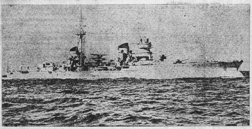
Este es el navío que trajo a su bordo al ministro de Negocios Extranjeros de Italia, conde Ciano. Construido en 1935, es hermano gemelo del "Emmanuele Filiberto Duca d'Abate" (1934). Desplaza 8.000 toneladas, tiene una eslora de 185,95 metros, 17,5 de manga y 4,98 de calado. Se construyó en los astilleros Ansaldo, de Génova, siendo Puesto en grada en 1932. La potencia de máquinas es de 110.000 c. v., que desarrollan una velocidad máxima de 365 millas horarias, distribuyéndose su centro generador motriz en dos turbinas: Parsons y Belluzo, que mueven dos hélices, poseyendo seis calderas Yarrow y cargando 1.200 toneladas de mazout. La tripulación está compuesta por 25 oficiales y 500 hombres. Y el armamento por ocho piezas de 152 mm., seis de 100, ocho de 37 A. A., y contando el crucero con una protección de una cintura de 120 mms. Finalmente, hay que hacer constar que las piezas de 152 mms. tienen un alcance máximo de 27 a 29.500 metros, con proyectiles de 49 kgs, y una velocidad normal de tiro de cuatro a cinco disparos por minuto.
