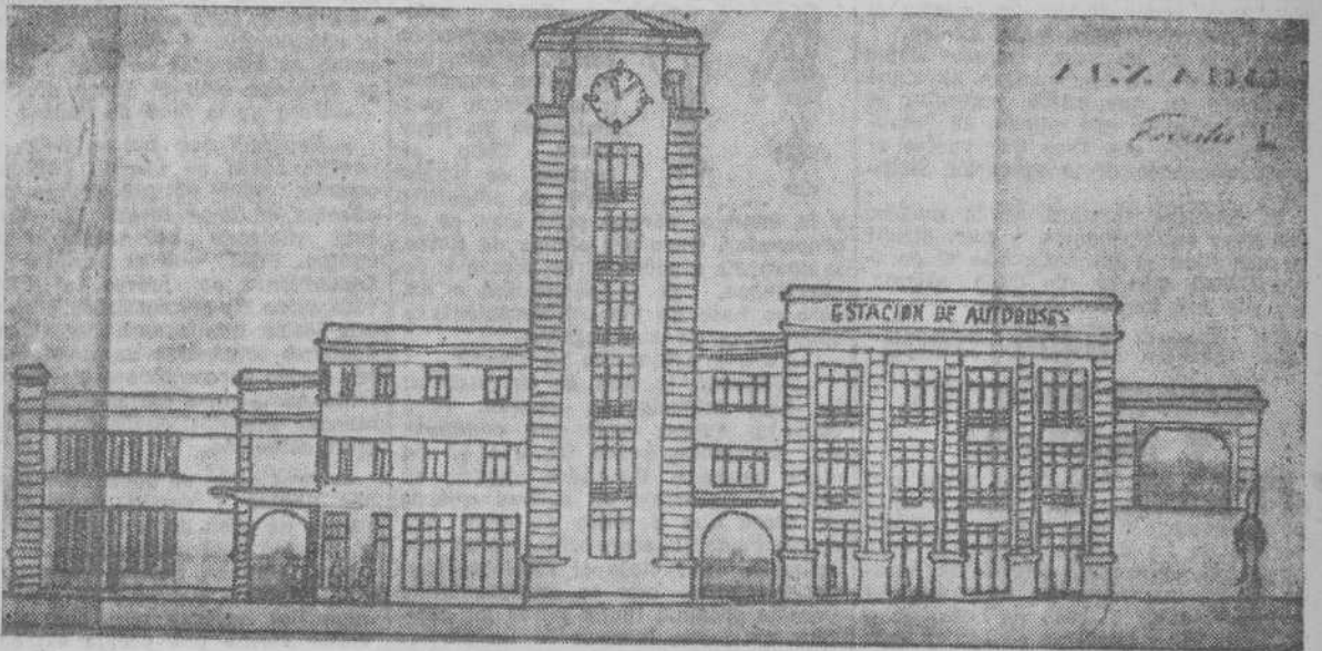
FACHADA PRINCIPAL DE LA PROYECTADA ESTACION DE AUTOBUSES
