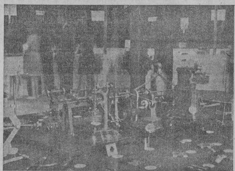
Torno de relojero, que puede contemplarse en funcionamiento, presentado por la Maestranza de Artillería
