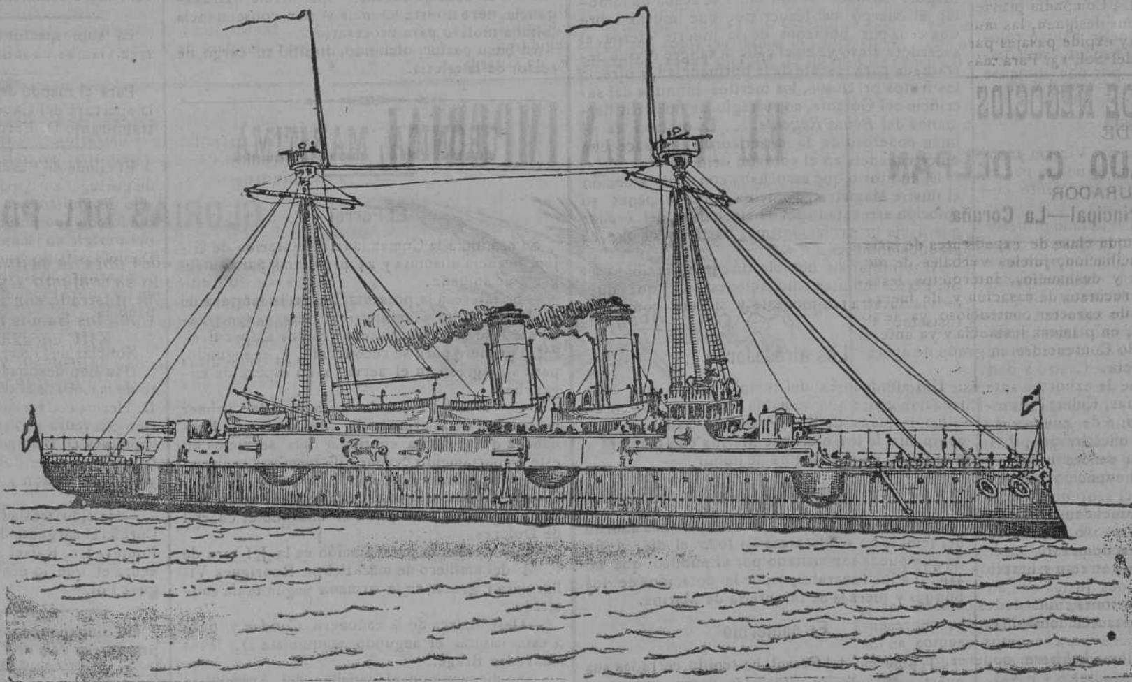
El Reina Regente fué construido en Inglaterra por la casa Thompson de Glasgow y botado al agua en el año 1887.—Prestó servicio por más de siete años.—El casco era de acero, con un desplazamiento de 4.770 toneladas.—Sus dimensiones eran eslora 97'3 metros, manga 15'43 y puntal 8'92.—El calado máximo en su línea de agua era de 6,50 metros.—Tenía dos máquinas gemelas de triple expansión, dos hélices y cuatro calderas dobles con una fuerza de 11.598 caballos indicados; era un buque de mucho andar que podía alcanzar en casos extraordinarios y sostener bastante tiempo, una marcha de 20 millas por hora.—Tenía una cubierta protectora de 120 milímetros de espesor, numerosos compartimientos estancos y unos tanques ó depósitos que, llenos de agua, aumentaban la estabilidad del buque sirviendo de lastre.—Su artillería la componían cuatro cañones González Hontoria de 24 centímetros, montados en cubierta, dos á popa y dos á proa; seis de 12 centímetros, del mismo autor; seis Nordenfeld de 57 milímetros y otro de 42; dos cañones revolver Holtchiss de 37 milímetros; dos ametralladoras Nordenfeld de 11 milímetros; cuatro de tiro rápido Holtchiss de 37, y dos de 7 centímetros González Hontoria.—Montaba además 5 tubos de lanzar torpedos y dos cofas militares.—El Reina Regente ha tenido cinco comandantes que fueron los capitanes de navío siguientes: D. Vicente Montojo, D. Ismael Warleta, D. José Pilon, D. José Pareles y D. Francisco Sanz de Andino que había tomado el mando el 20 de Noviembre del 94 es decir cuatro meses antes de la catástrofe ocurrida el 10 de Marzo.—Su dotación reglamentaria era en total de 430 hombres.
