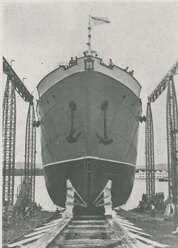
Buque bacaladero SANTA CECILIA , de 2.500 toneladas para P. E. B. S. A., preparado para lanzamiento
