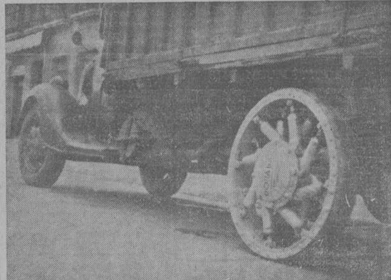
BARCELONA.—Rueda sustitutiva de los neumáticos, construida a base de acero y contrachapado de madera, cuyas pruebas oficiales se han realizado en Monjuich el pasado domingo. (Foto CIFRA).
