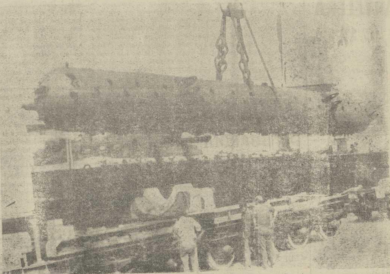
TARRAGONA. — Elemento de 280 toneladas de peso procedente de Estados Unidos y que ha sido desembarcado en esta ciudad, con destino a la central nuclear que se está construyendo en Teruel. (CIFRA GRAFICA.)
