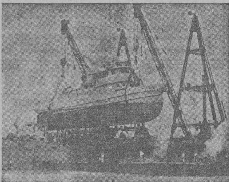
Un buque de 185 toneladas, del tipo "Liberty", botado al agua en Nueva Orleans por el nuevo procedimiento que muestra la foto; es decir, descolgado al agua con un par de grúas. El navío se destinará al envío de suministros a China por parte de la UNRRA.
