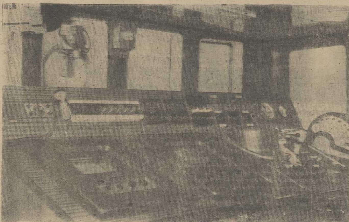
La mesa del puente del "Mar de Galilea", instalada por "RADIONAVAL", un alarde de técnica y funcionalidad.
