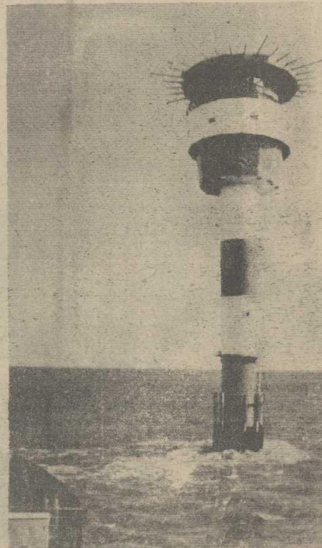
NURNBERG. — Buques faro, que han de ser atendidos necesariamente por personal especializado, son relevados cada vez más por faros automatizados. En el faro de la fotografía, que muestra el camino a los buques en el Mar del Norte, se instalaron tres grupos electrógenos. Están equipados para el funcionamiento completamente automático con telecontrol desde tierra.
