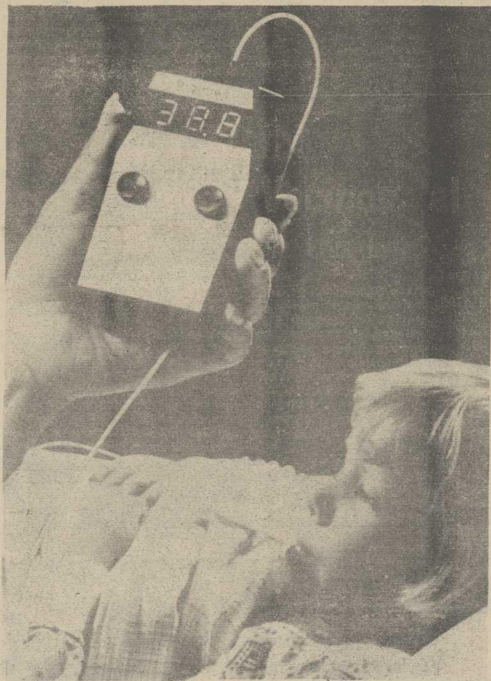
MUNICH. — La medición de la temperatura corporal se efectúa más agradablemente para el paciente y con mayor rapidez para el personal sanitario con ayuda de este nuevo termómetro clínico electrónico. De "sensor" sirve un termoconductor fabricado por la Siemens en la República Federal de Alemania, un elemento que modifica su resistencia eléctrica ante la mínima oscilación de la temperatura.
