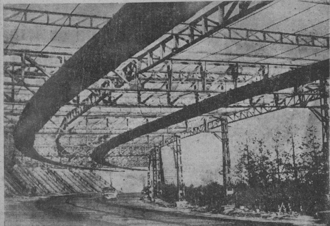
La carretera japonesa de Tokio a Yokohama cruza un importante y frecuentado terreno de golf. Continuamente las pelotas del juego caían a la carretera para los automóviles y, especialmente, para los motoristas. Una red de tela metálica preserva ahora el camino. Estas gigantescas construcciones metálicas sirven además de puente sobre la carretera.
