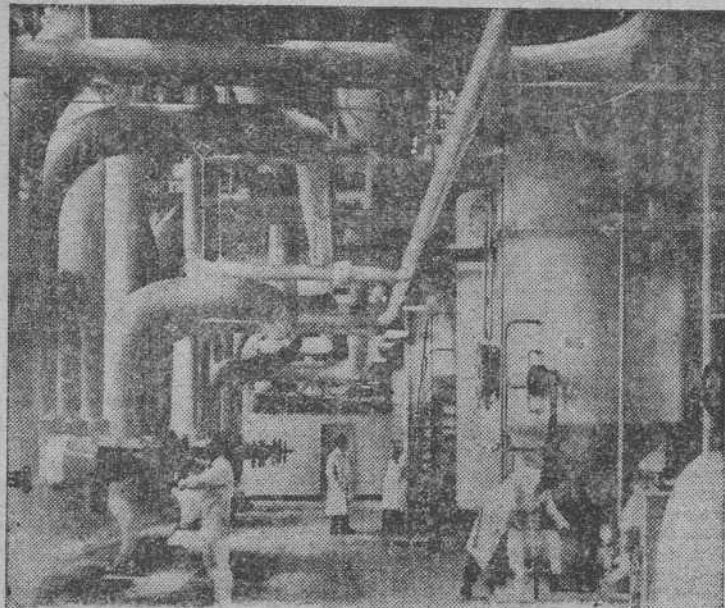
Sala de turbinas de la central nuclear de Calder Hall. En esta central está inspirada la que un grupo industrial italiano ha contratado en Inglaterra para su instalación en el Norte de Italia.
