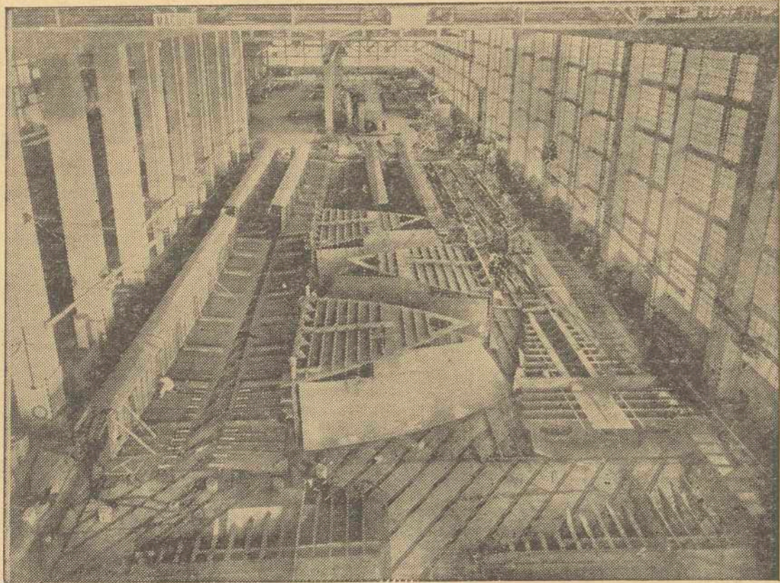
Prefabricado de buques en el taller de herreros de ribera
