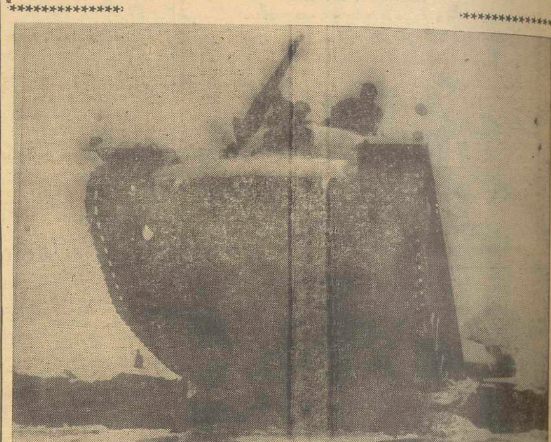
El nuevo carro de combate proyectado y fabricado íntegramente en Suiza, el «Pz 61» durante las pruebas que ha realizado en público ante la prensa, la radio y la televisión en el polígono de Thun. Armado con un cañón de 105 milímetros y otro de 20 milímetros con una cadencia respectiva de 1.000 y 800 disparos por minuto, pesa unas 35 toneladas y goza de una impresionante maniobrabilidad. (FOTOFIEL)
