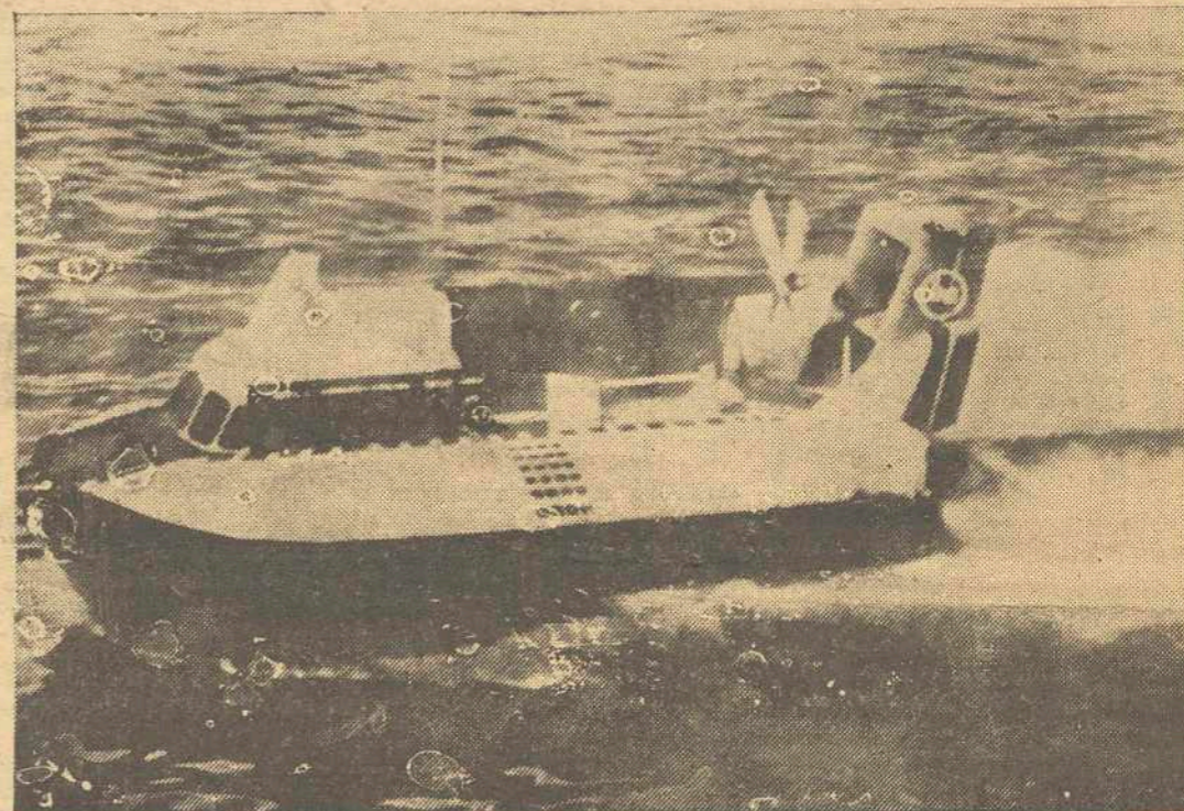
He aquí una versión norteamericana del vehículo de invención británica, e. Hovercraft. La foto fue tomada durante las pruebas realizadas por la moderna embarcación sobre el río Potomac, Washington. El vehículo tiene 39 pies de largo y desplaza 9 toneladas. — (Foto AP LOGOS)
